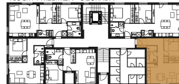
TLOCRT PRIZEMLJA - C ZGRADA
