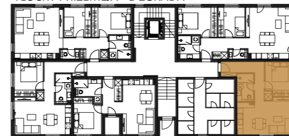
TLOCRT PRIZEMLJA - B ZGRADA
